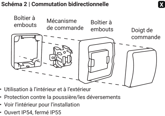
Schéma 1 | Interrupteur va-et vient Schéma 2 | Commutation bidirectionnelle
